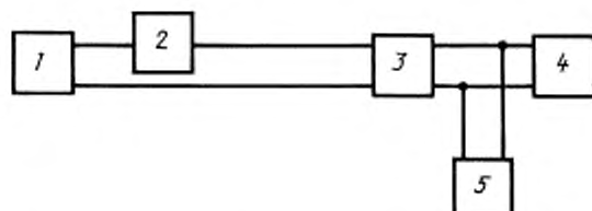
1 — испытуемый ТА; 2 — миллиамперметр постоянного тока; 3 — питающий комплект; 4 — генератор сигналов низкочастотный; 5 — электронный вольтметр переменного напряжения
