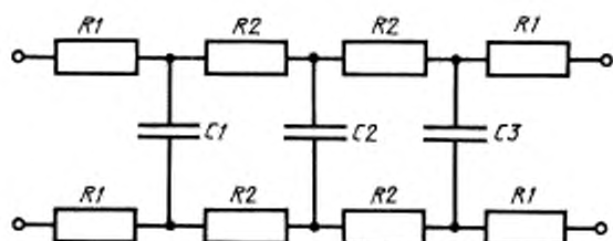
R1 — резистор с сопротивлением (52,5 \pm 0,5) Ом; R2 — резистор с сопротивлением (105 \pm 1) Ом; C1 — C3 — конденсаторы емкостью (55,0 \pm 0,3) нФ
