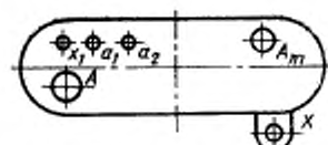
б) автотрансформатор АОДЦТН-417000/750/500
