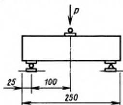
Схема испытания кирпича на изгиб
