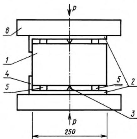
Схема раскладывания кирпича в прессе
