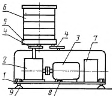
1 — плита; 2 — редуктор; 3 — электродвигатель; 4 — эксцентрик; 5 — диск; 6 — комплект сит; 7 — ручка управления; 8 — уровень; 9 — винт регу- лировочный
