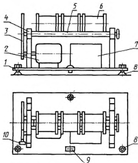
1 — плита; 2 — электродвигатель; 3 — привод; 4 — стойка; 5 — валки; 6 — барабаны; 7 — пульт управления; 8 — шнур регулировочный; 9 — уровень; 10 — ручка
