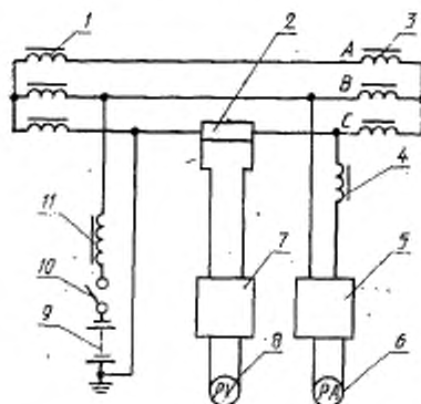
1 — питающий трансформатор; 2 — шунт; 3 — измеряемая обмотка; 4 — индуктивность; 5 — фильтр; 6 — микроамперметр; 7 — фильтр; 8 — аккумуляторная батарея; 9 — выключатель; 10 — дроссель
