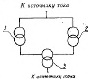
1 — испытуемый трансформатор; 2 — вспомогательный трансформатор; 3 — промежуточный трансформатор
