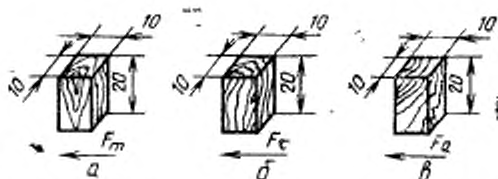
а—нагрузка, истирающая образец по торцовой поверхности ( F_m ) ( F_T ); б—нагрузка, истирающая образец по тангентальной поверхности; а—нагрузка, истирающая образец по радиальной поверхности ( F_a )
