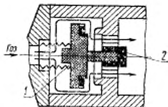
1 — пружина сжатия; 2 — плавкий элемент (например расплавляющийся при- пой)
