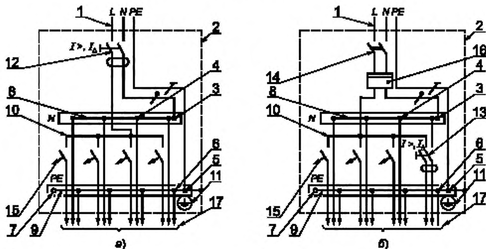
Рисунок А.1 — Схемы квартирных щитов (группового и учетно-группового), присоединенных к распределительным цепям, отходящим от: а) этажного учетно-распределительного щитка; б) этажного распределительного щитка
