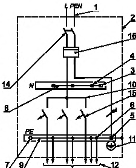
Рисунок А.1 — Схемы квартирных щитов (группового и учетно-группового), присоединенных к распределительным цепям, отходящим от: а) этажного учетно-распределительного щитка; б) этажного распределительного щитка
