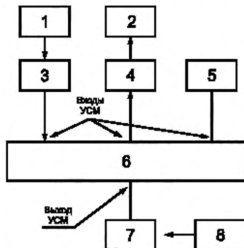
1 — генератор сигналов ВЧ, 2 — селективный микрометр; 3, 4 — согласованные коаксиальные переходы; 6 — УСМ; 5, 7 — согласованные экранированные нагрузки; 8 — миллиметр ВЧ
