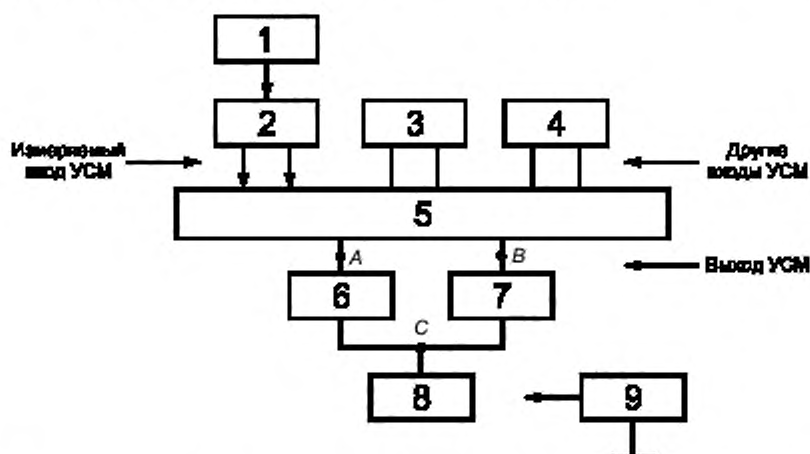
1 — генератор сигналов ВЧ; 2 — симметрирующее устройство; 3, 4 — согласованные нагрузки; 5 — УСМ; 6, 7 — несимметричные нагрузки с волновым сопротивлением, равным половине волнового сопротивления подключаемого фидера ( W/2 ); 8 — несимметричная нагрузка с волновым сопротивлением, равным четверти волнового сопротивления подключаемого фидера ( W/4 ); 9 — милливольтметр ВЧ
