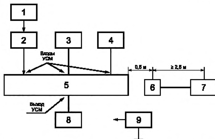
1 — генератор сигналов ВЧ; 2 — согласованный коаксиальный переход; 3, 4 — экранированные согласованные нагрузки; 5 — УСМ; 6 — измерительная антенна; 7 — измеритель напряженности ЭМП; 9 — милливольтметр ВЧ
