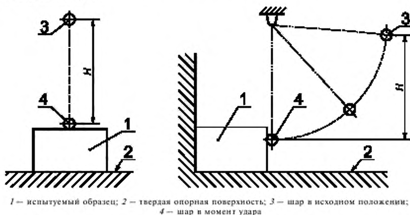
Рисунок 1 — Испытания на удар с помощью стального шара
