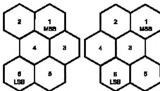
Рисунок 1 — Модули типичного знака символа в символе MaxiCode
