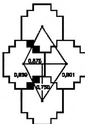
Рисунок J.5 — Вложенная структура модулей MaxiCode при разрешении 8 точек/мм
