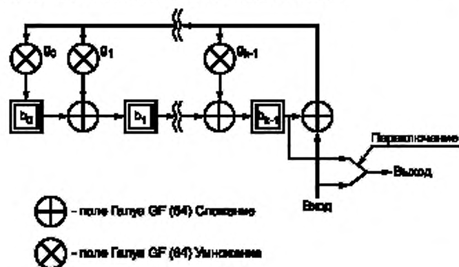
Рисунок 7 — Схема кодирования кодовых слов коррекции ошибок
