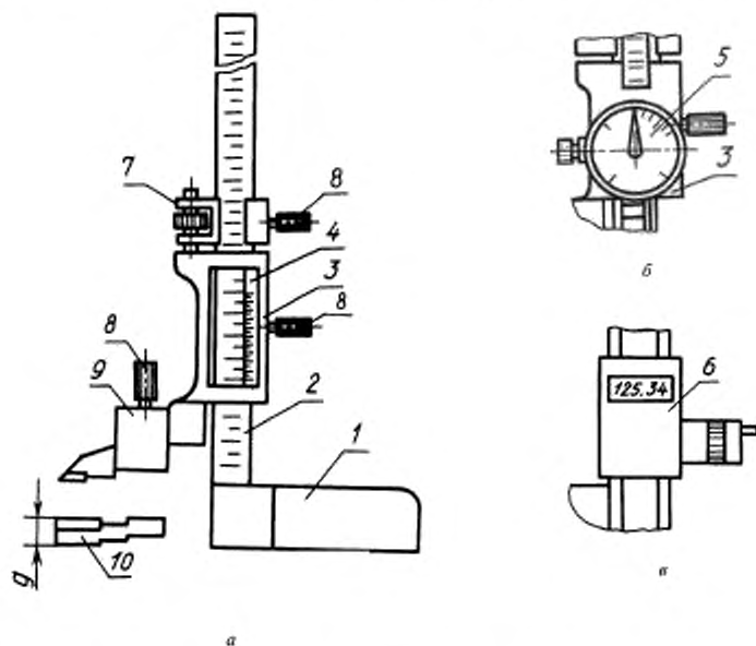
1 — основание; 2 — штанга; 3 — рамка; 4 — нониус; 5 — круговая шкала; 6 — цифровое отсчетное устройство; 7 — микрометрическая подача; 8 — стопорные винты; 9 — разметочная ножка; 10 — измерительная ножка
