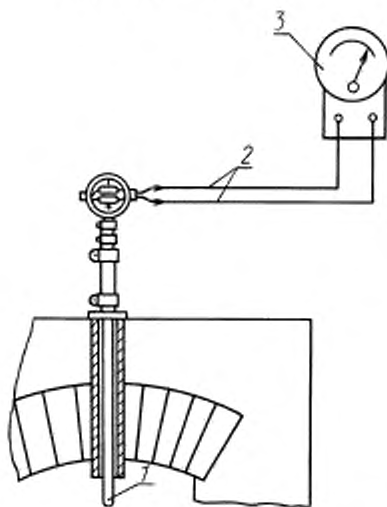
Схема установки термопары
