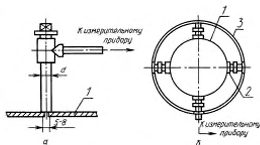
1 — стенка газохода; 2 — патрубок; 3 — соединительный трубопровод
