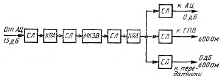
Типовой тракт первичного распределения программ звукового вещания с магистральным или внутризоновым каналом звукового вещания
