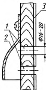
1 — вентиляционные отверстия; 2 — металлический козырек; 3 — водонепроницаемый материал
