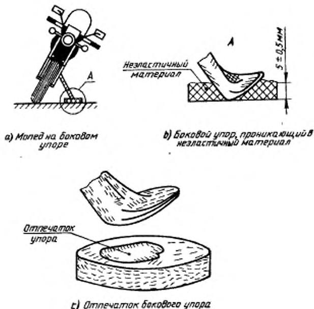
Рисунок 1 — Боковой упор
