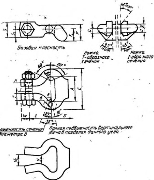
Рисунок 1 — Соединительное звено
