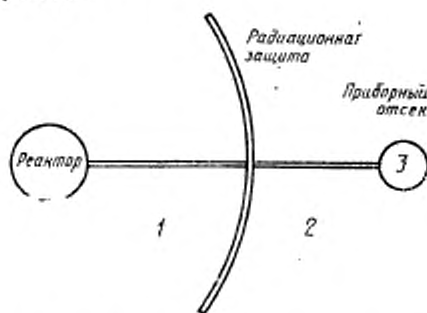
Рисунок 1 — Схема космического аппарата с бортовым ядерным реактором
