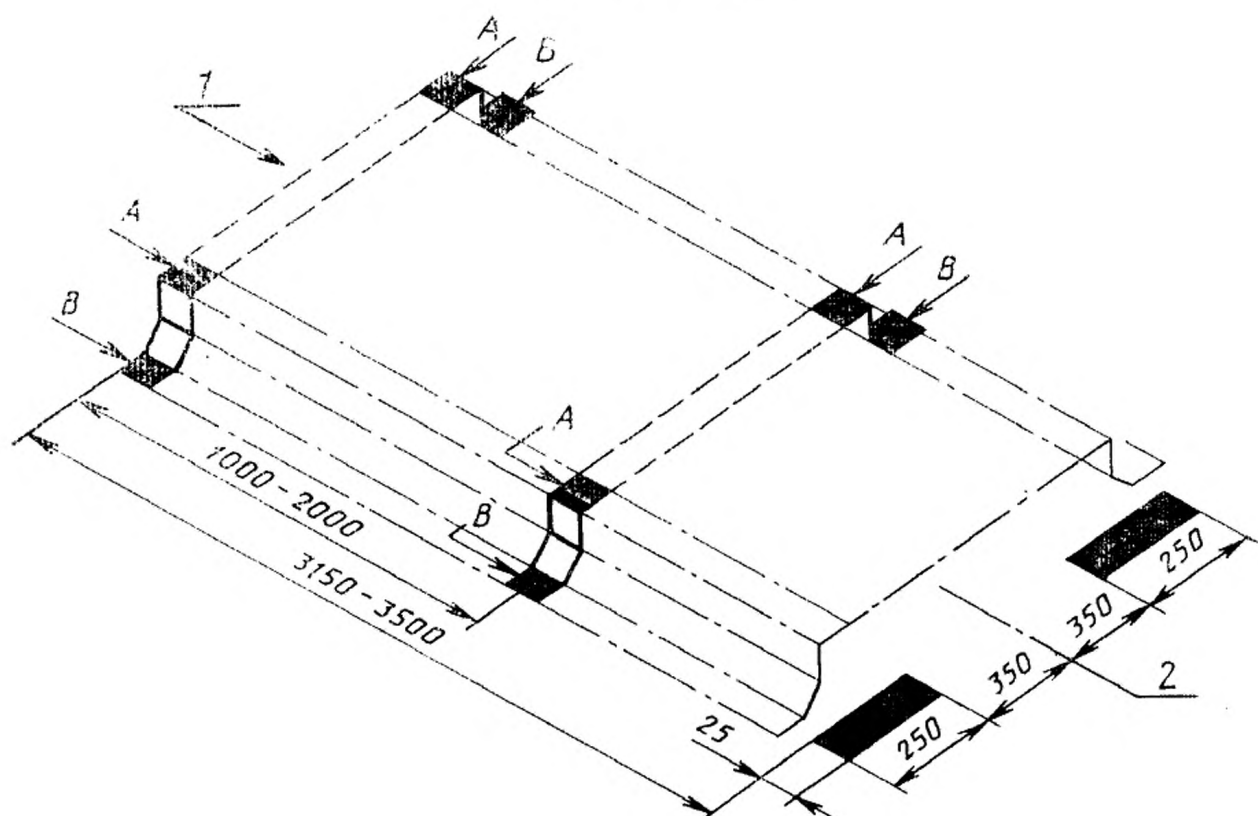
1 — торец контейнера; 2 — центральная ось Рисунок Б/10
