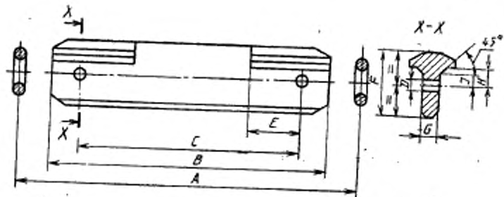
Рисунок 1 — Размеры Т-образных скребков
