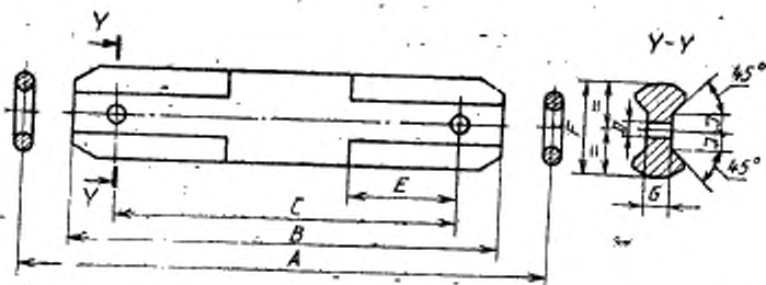
Рисунок 2 — Размеры I-образных скребков
