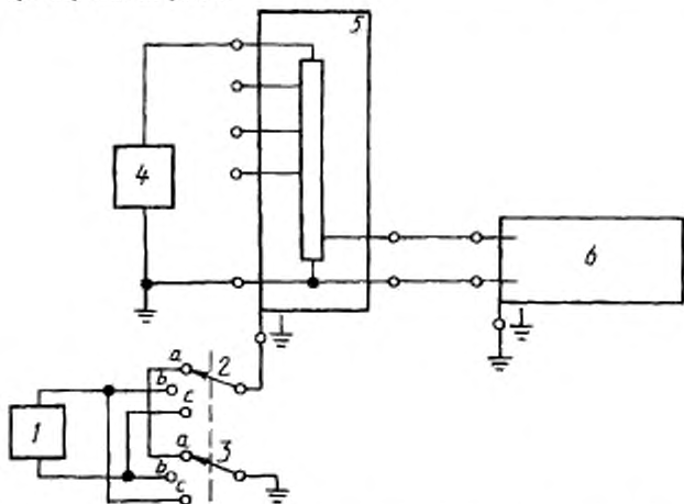
1 — источник напряжения постоянного тока помехи общего вида; 2, 3 — двухполюсный, трехпозиционный выключатель; а — выключение и короткое замыкание; б — прямое напряжение помехи общего вида; с — обратное напряжение помехи общего вида; 4 — источник номинального входного напряжения постоянного тока; 5 — испытуемый делитель напряжения; 6 — потенциометр постоянного тока
