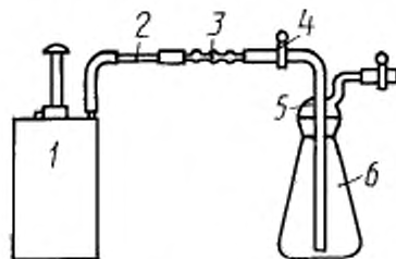
1 — газопровод УГ-2; 2 — индикаторная трубочка; 3 — фильтрующий патрон; 4 — зажимы пружинящие; 5 — пробка-насадка Дрекслея; 6 — колба коническая
