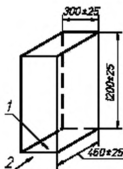
Рисунок 1 – Металлическая камера
