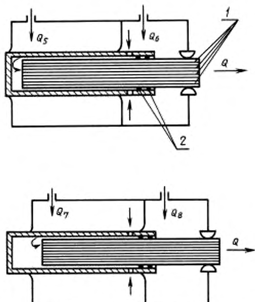
1 — микрокапиллярный калибр перепада давления; 2 — уплотнительные кольца
