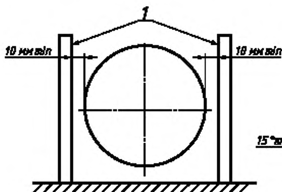
Рисунок 106 — Защита барабанов
