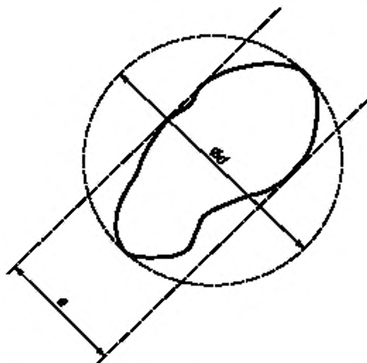
Рисунок AA.1 — Определение стандартного отверстия
