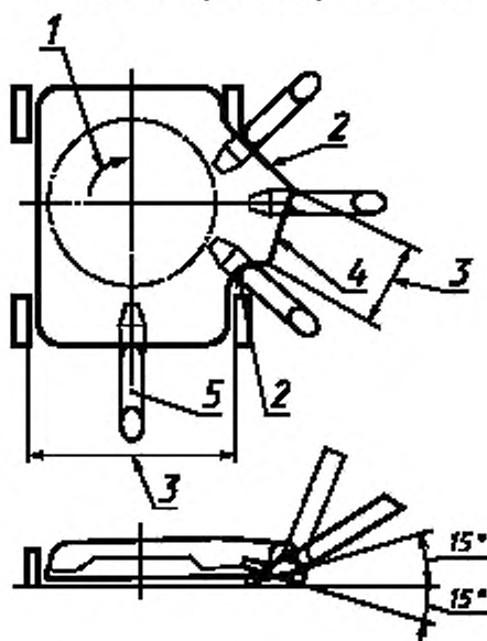
Расположение пробника при испытании
