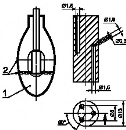
Рисунок 7 — Распылитель
