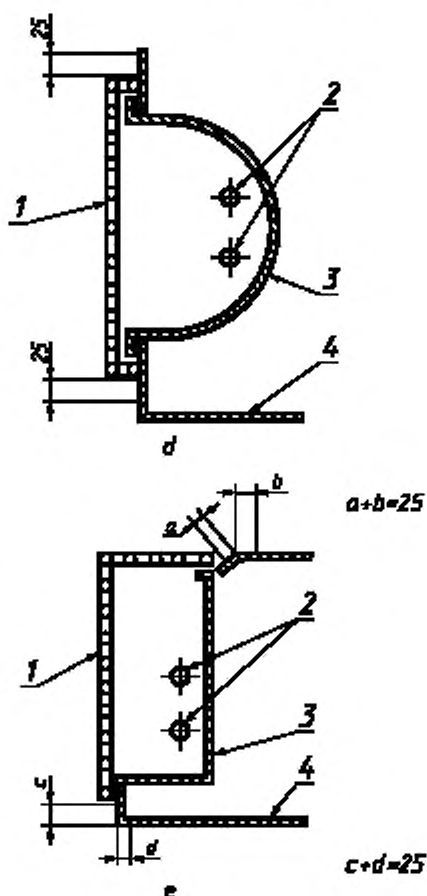
1 — каминная решетка; 2 — нагревательные элементы накаливания; 3 — рефлектор; 4 — корпус
