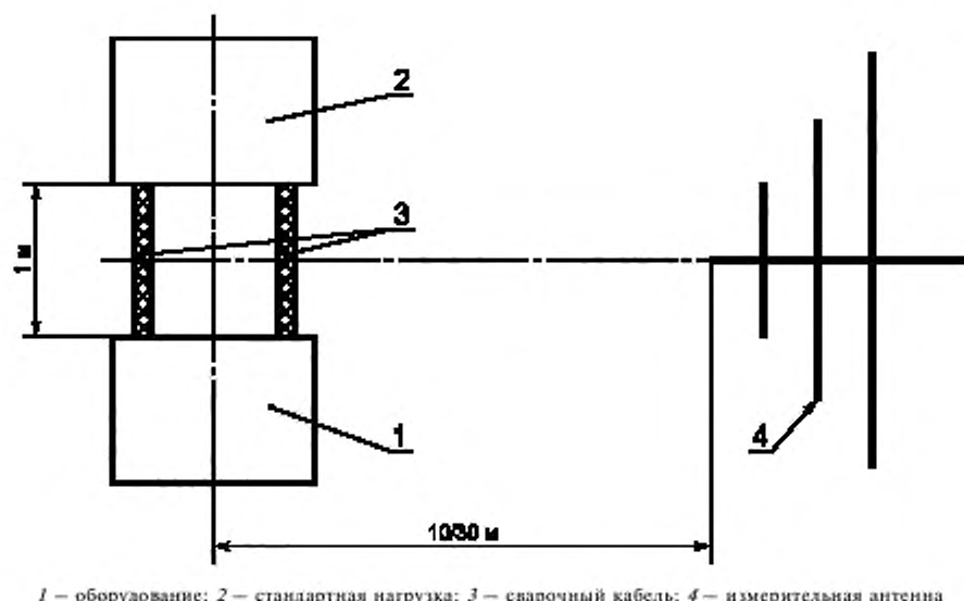
Рисунок 2 — Расположение сварочного оборудования и стандартной нагрузки по отношению к антенне
