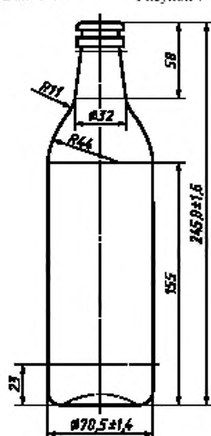
Номинальная вместимость, см 3 , — 544. Полная вместимость, см 3 , — 575 ± 15.
