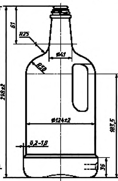
Рисунок 25 — Бутылка типа XXV
