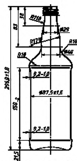
Рисунок 23 — Бутылка типа XXIII
