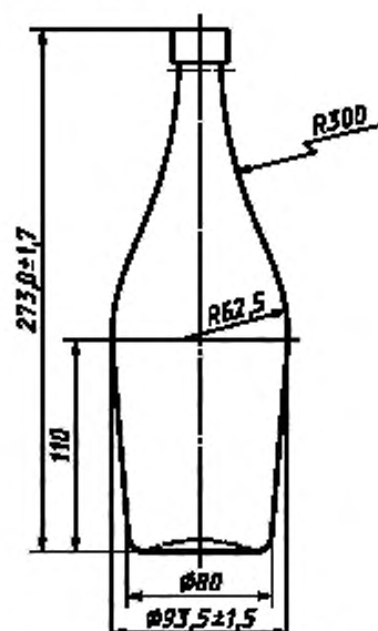
Рисунок 20 — Бутылка типа XX
