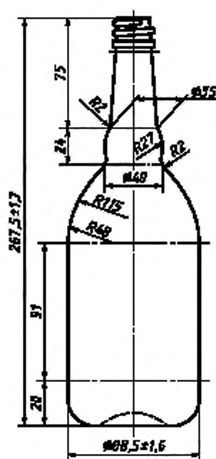
Номинальная вместимость, см 3 , — 700. Полная вместимость, см 3 , — 725 ± 15.
