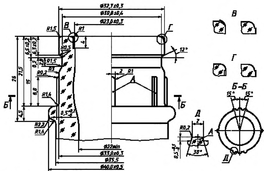
Рисунок 46 — Венчик типа КТМ-30
