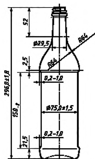
Рисунок 22 — Бутылка типа XXII
