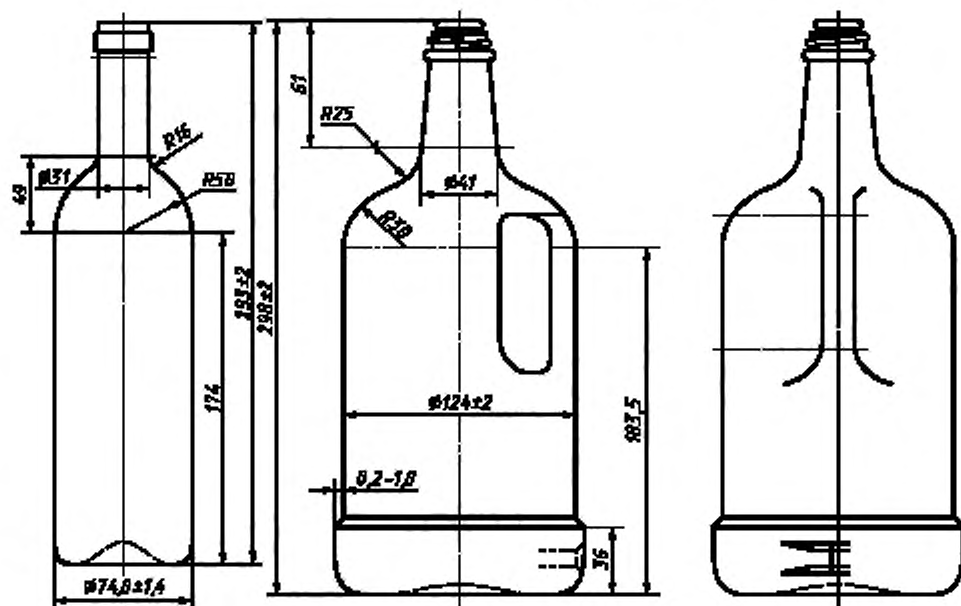
Рисунок 25 — Бутылка типа XXV
