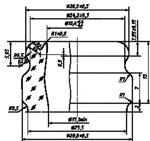
Контролируемые размеры венчика горловины: \varnothing 26,5 \pm 0,3 ; \varnothing 28,0 \pm 0,3 ; \varnothing 16,4^{+0,6}_{-0,4} должен быть на глубине до 3 мм от торца венчика; \varnothing 15,1 \text{ min} — в остальной части горловины. Допускается внутренний диаметр венчика 17,5 \pm 1,0 на глубине до 3 мм от торца венчика.
