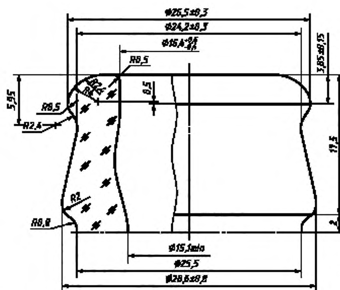
Контролируемые размеры венчика горловины: \varnothing 26,5 \pm 0,3 ; \varnothing 16,4^{+0,6}_{-0,4} должен быть на глубине до 3 мм от торца венчика; \varnothing 15,1 \text{ min} — в остальной части горловины. Допускается внутренний диаметр венчика 17,5 \pm 1,0 на глубине до 3 мм от торца венчика.
