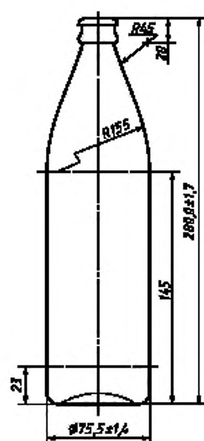
Номинальная вместимость, см 3 , — 775. Полная вместимость, см 3 , — 800 ± 15.
