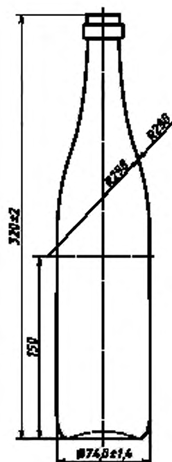
Рисунок 25 — Бутылка типа XXV
