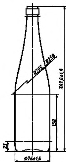
Номинальная вместимость, см 3 , — 700. Полная вместимость, см 3 , — 725 ± 15.
