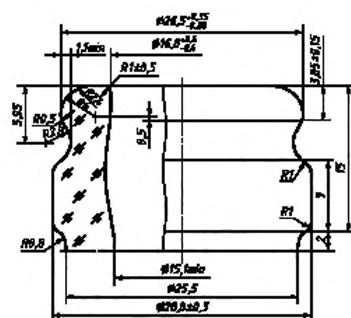
Контролируемые размеры венчика горловины: \varnothing 26,5^{+0,15}_{-0,20} ; \varnothing 28,0 \pm 0,3 ; \varnothing 16,0^{+0,6}_{-0,4} должен быть на глубине до 3 мм от торца венчика; \varnothing 15,1 \text{ min} — в остальной части горловины.
