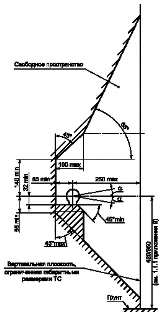
Рисунок 25а — Свободное пространство и размеры для (размещения) шарового наконечника, вид сбоку
