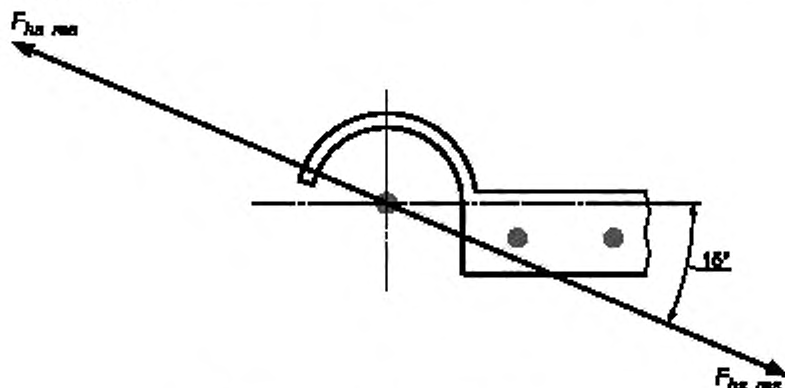
Рисунок 23 — Динамическое испытание
