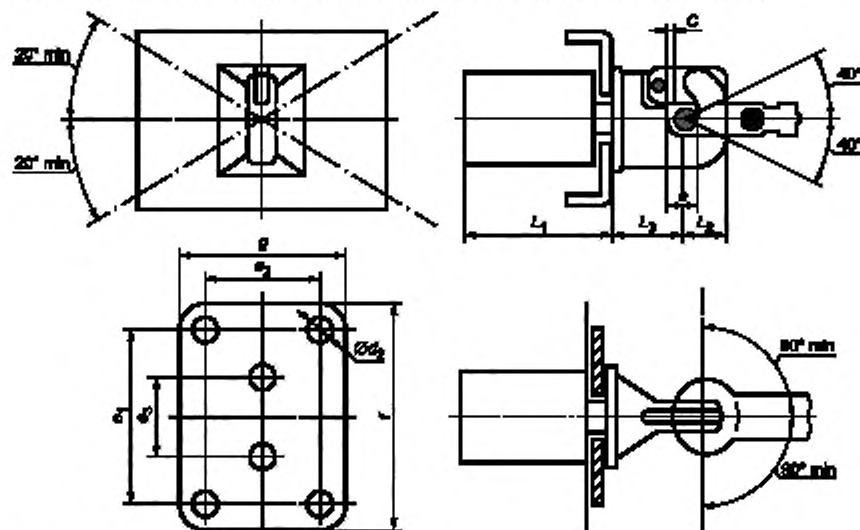
Рисунок 19 — Размеры и углы отклонения сцепных устройств типа «крюк-петля» класса K
