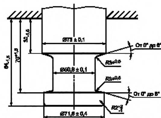
Рисунок 18 — Размеры шкворней седельно-сцепных устройств класса H50
