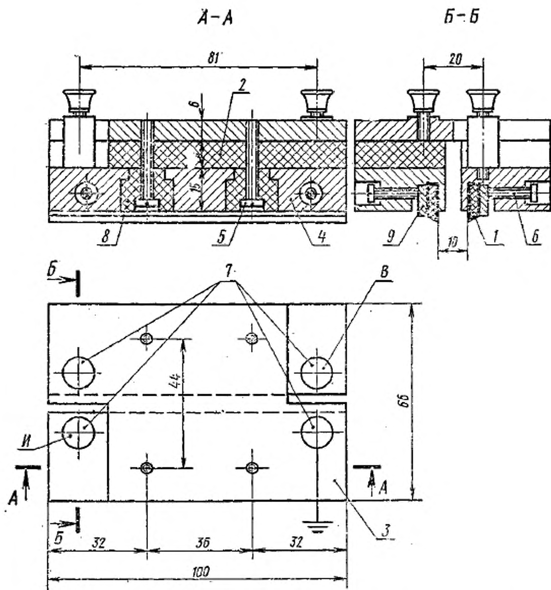
1—ножевые электроды (резина, обернутая фольгой); 2—прокладка; 3—основание; 4—электродные бруски; 5—винты для крепления; 6—прижимные винты; 7—клеммы; 8—втулки; 9—планки прижимные; B—электрод напряжения; И—измерительный электрод
