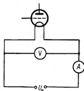
U_n — источник постоянного напряжения накала; V — вольтметр постоянного тока; A — амперметр постоянного тока
