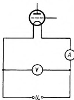
U_n — источник постоянного напряжения накала; A — амперметр постоянного тока; V — вольтметр постоянного тока
