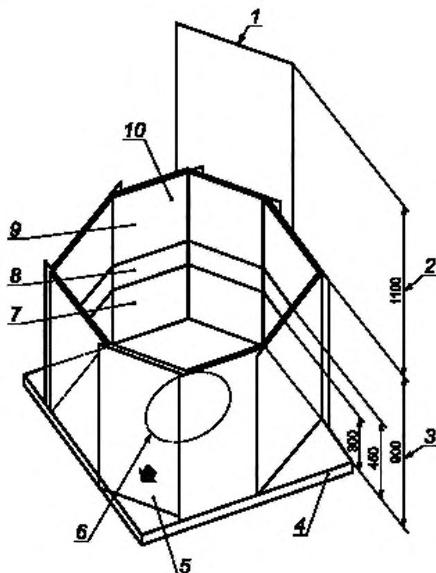
1 — верхняя зона оператора; 2 — дополнительная зона (одинарная толщина крафт-бумаги); 3 — общая высота панели-мишени; 4 — основание (рисунок ВВ.1); 5 — передняя сторона; 6 — подвижная зона; 7 — нижняя зона; 8 — средняя зона; 9 — верхняя зона; 10 — титовая панель-мишень (рисунок АА.3)
