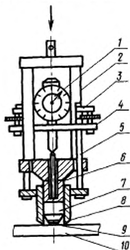
1 — индикатор; 2 — стойка; 3 — регулировочный винт; 4 — планка; 5 — колодка; 6 — нижний направляющий; 7 — основание; 8 — держатель для шарика; 9 — шарик; 10 — образец
