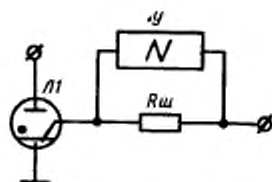
Л1 —испытываемый игнитрон; У —осциллограф; R_{ш} —резистор
