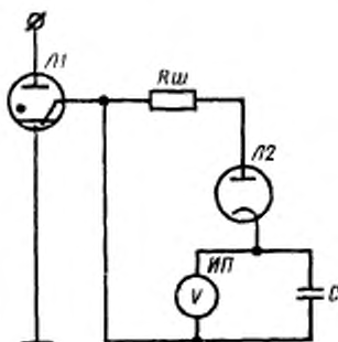
Л1 — испытываемый икитрон; Л2 — неонитрон; ИП — вольтметр; С — конденсатор; Rш — резистор
