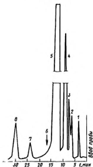
Типовая хроматограмма технического этилацетата
