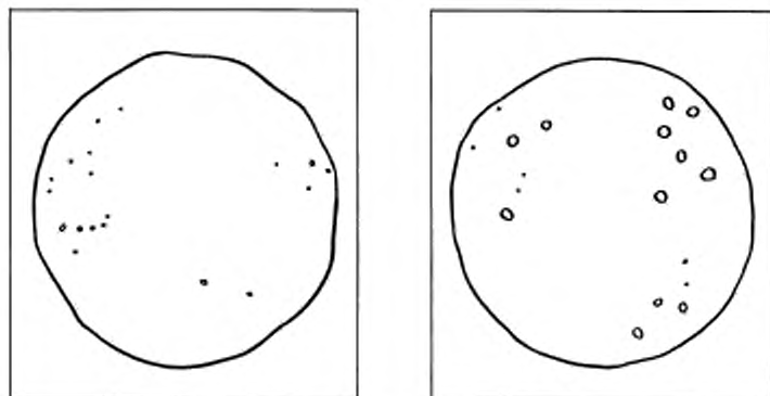
Лепешки, выдержавшие испытания на равномерность изменения объема
