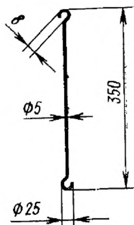
Удлинительная штанга
