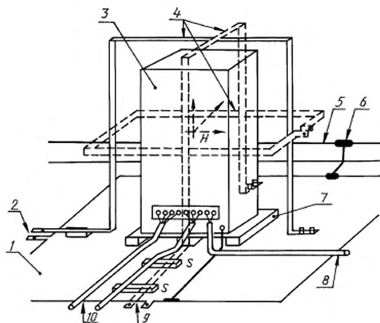
1 — плоскость заземления; 2 — к ИГ; 3 — ИТС; 4 — индукционная катушка; 5 — защитное заземление; 6 — соединение плоскости заземления с целью защитного заземления; 7 — изолирующая опора; 8 — к сети электропитания; 9 — к ИГ; 10 — к источнику сигналов (имитатору)
