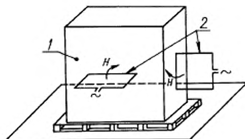
1 — ИТС; 2 — индукционная катушка
