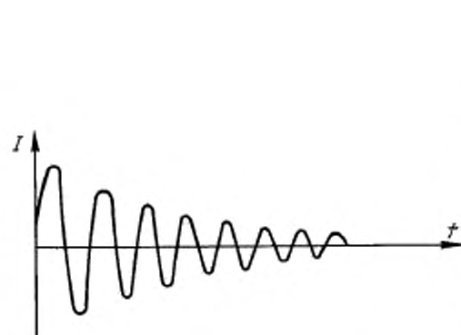
Рисунок 2 — Форма выходного тока ИГ
