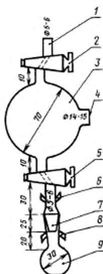
1 — отрезок, 2, 5 — одноходовые краны; 3 — емкость для сбора «летучих» (100—120 см 3 ); 4 — отверстие для самозатягивающейся пробки; 6, 8 — усики; 7 — шлиф № 14—14,5 мм; 9 — колба со шлифом (№ 14—14,5 мм) для латекса
