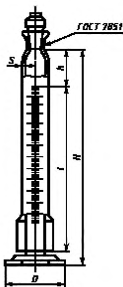
Исполнение 4а (с пластмассовой пробкой и пластмассовым основанием)
