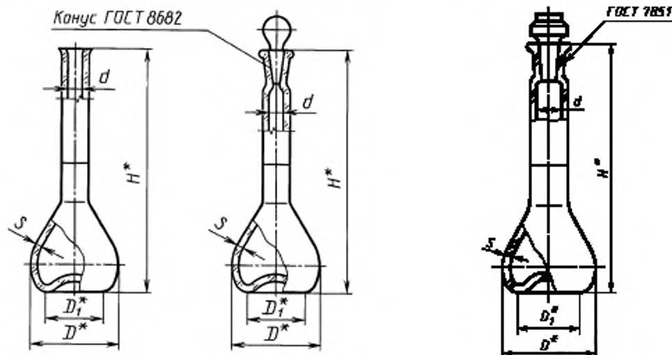
Исполнение 2а (с одной отметкой и пластмассовой пробкой)
