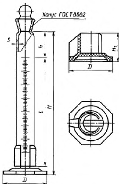
Исполнение 4 (с припильной пробкой и пластмассовым основанием)
