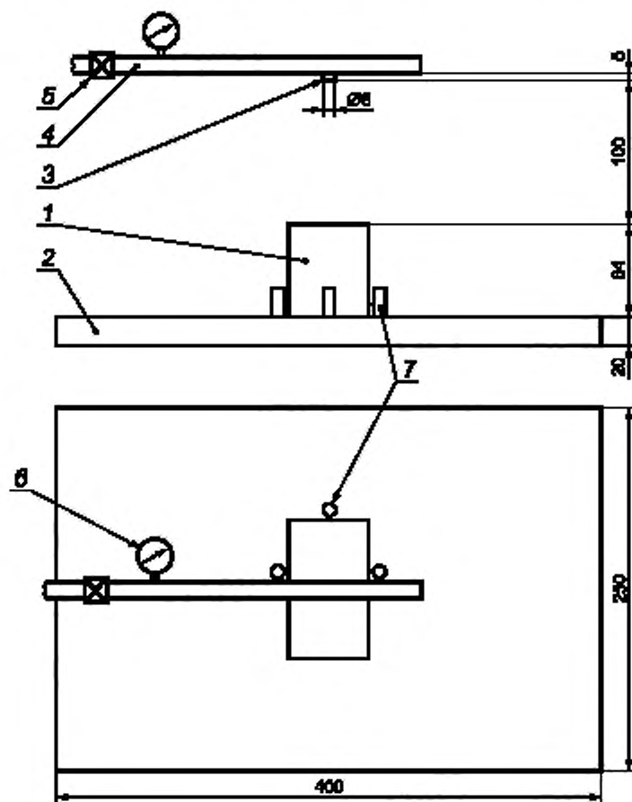
Рисунок А.1 — Общий вид плиты и устройства для охлаждения
