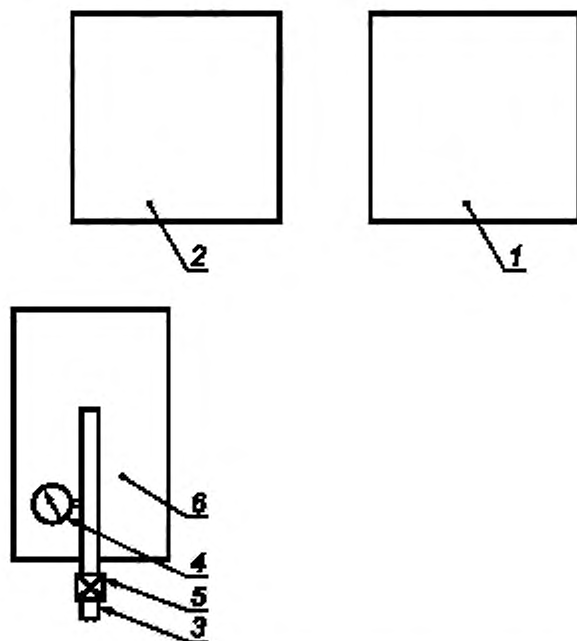
Рисунок Б.1 — Схема расположения испытательного оборудования
