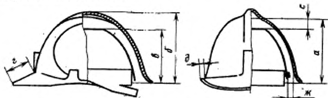
а—высота корпуса без учета ребра жесткости; б—высота корпуса с ребром жесткости; в—глубина внутренней оснастки; с—ширина козырька; д—ширина полей; ж—вертикальный безопасный зазор; ж—кольцевой зазор.
