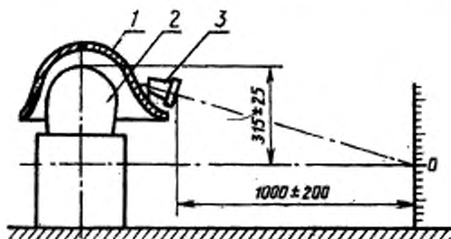
1 — каска; 2 — макет головы; 3 — фара светильника Черт. 2
