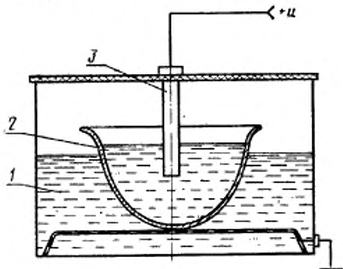
1—электрод; 2—корпус каски; 3—подающий электрод
