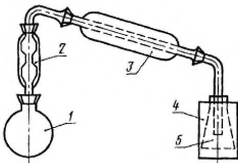
1 — круглодонная колба; 2 — изгиб; 3 — холодильник; 4 — аллонж; 5 — цилиндр
