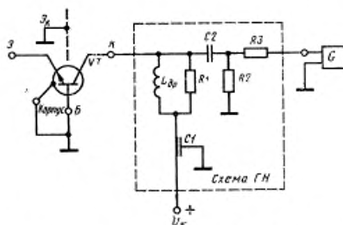
VT—измеряемый транзистор; Экран—экран в контактодержателе между выводами эмиттера и коллектора; C2—разделительный конденсатор; R2, R3—резисторы для развязки генератора сигналов; G—генератор сигналов; Lдp—дроссель для задания напряжения на коллектор транзистора; R1—резистор для подавления паразитного возбуждения транзистора; C1—блокировочный конденсатор.
