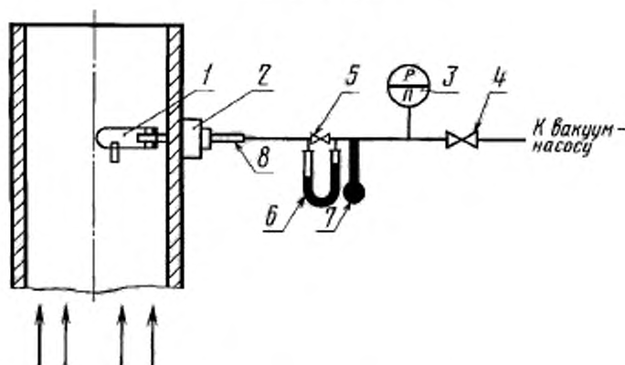
Схема отбора проб
