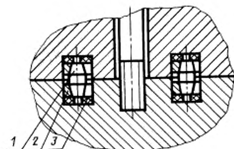
1 — фиксирующий палец; 2 — штулка разрезная; 3 — шайба упругая
