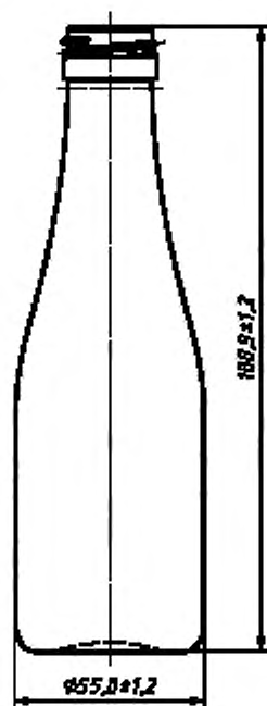
Венчик горловины — тип В-28Д. Номинальная вместимость, см 3 , — 200. Полная вместимость, см 3 , — 215 \pm 6 .
