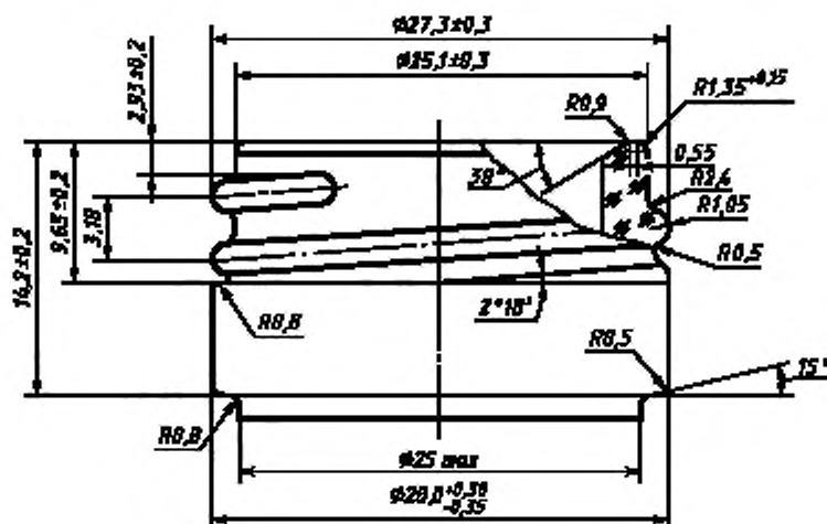
Рисунок 13 — Венчик типа В-28Д
