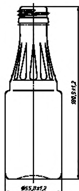
Венчик горловины — тип В-28Д. Номинальная вместимость, см 3 , — 200. Полная вместимость, см 3 , — 220 \pm 6 .
