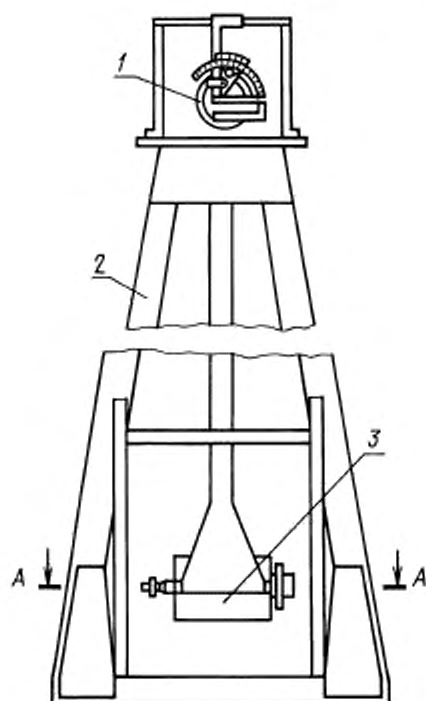
1 — угольник; 2 — рама; 3 — мортира
