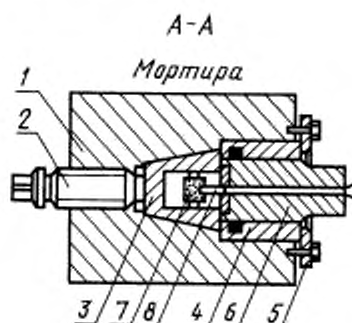
1 — корпус мортира; 2 — выжимной винт; 3 — взрывная камера; 4 — расширительная камера; 5 — фланец; 6 — снаряд; 7 — заряд ВВ; 8 — ЭД
