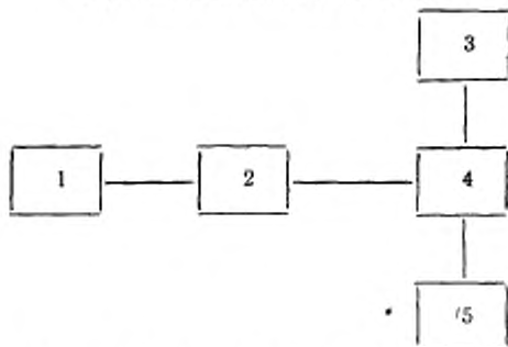
Схема соединения приборов при использовании образцового импульсного вольтметра
